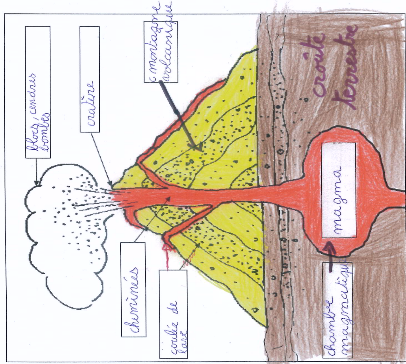
Schéma d'un volcan en coupe
